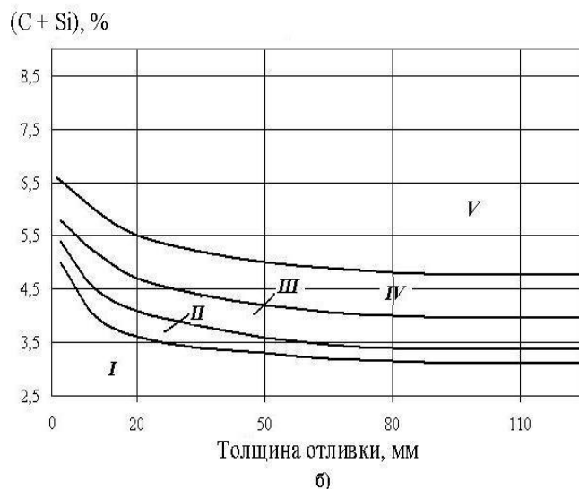
Рис. 1. Структурная диаграмма чугунов:
